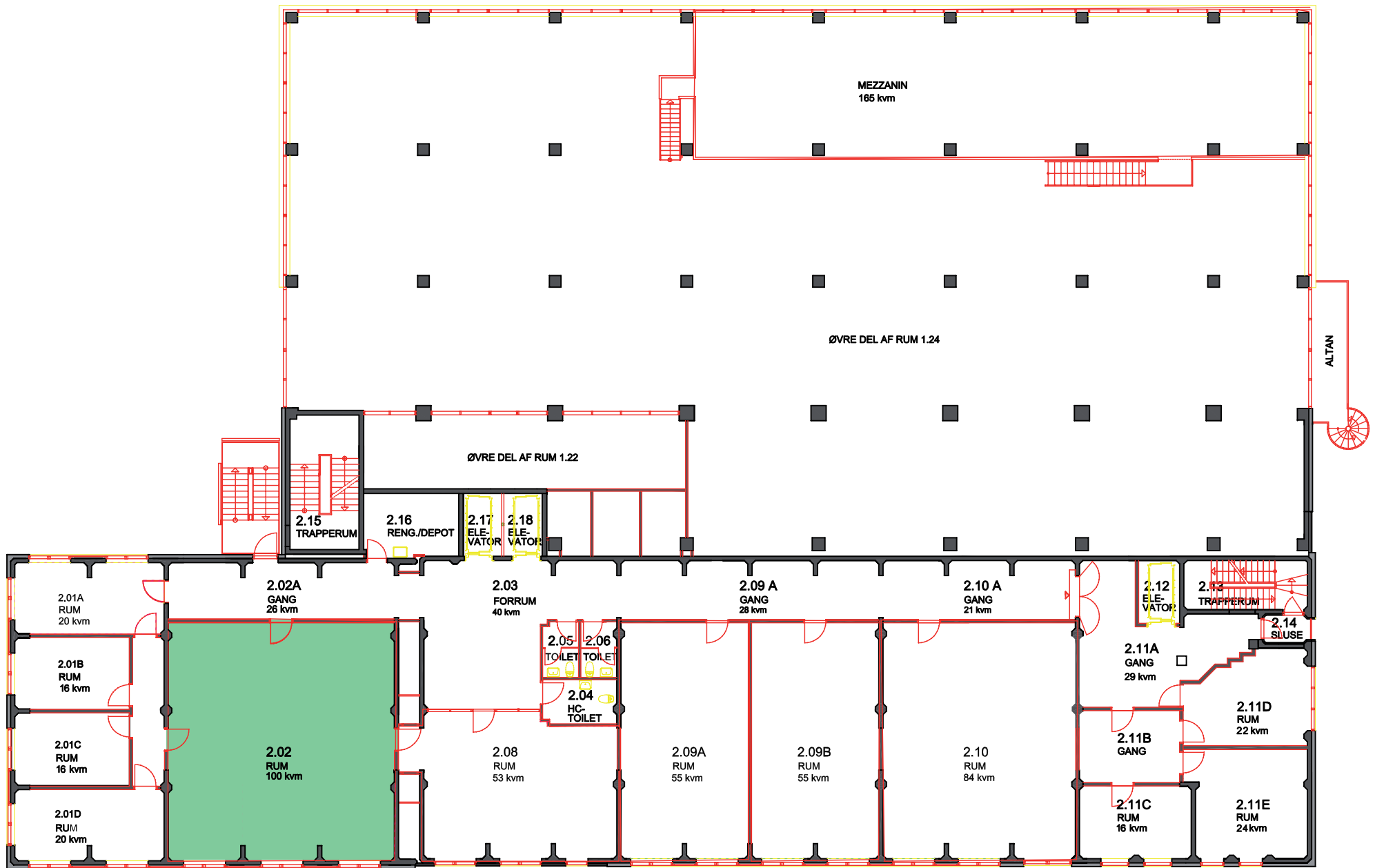
KATTEGAT SILO 1A + 2. SALS PLAN
